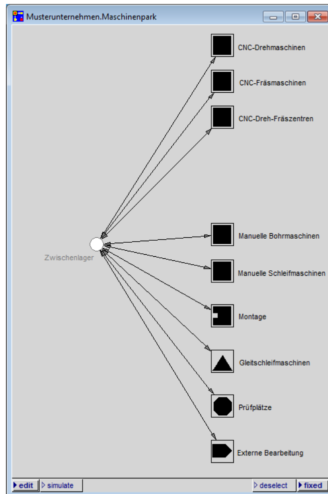
Abbildung 72: 2. Objektebene des Simulationsmodells Musterunternehmen
