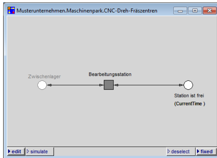
Abbildung 47: Angepasste Kategorie CNC-Dreh-Fräszentren
