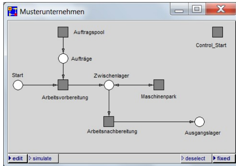
Abbildung 71: 1. Objektebene des Simulationsmodells Musterunternehmen
