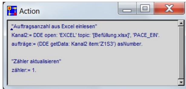
Abbildung 84: „Auskommentierte“ umgangssprachliche Erläuterung von Codefragmenten
