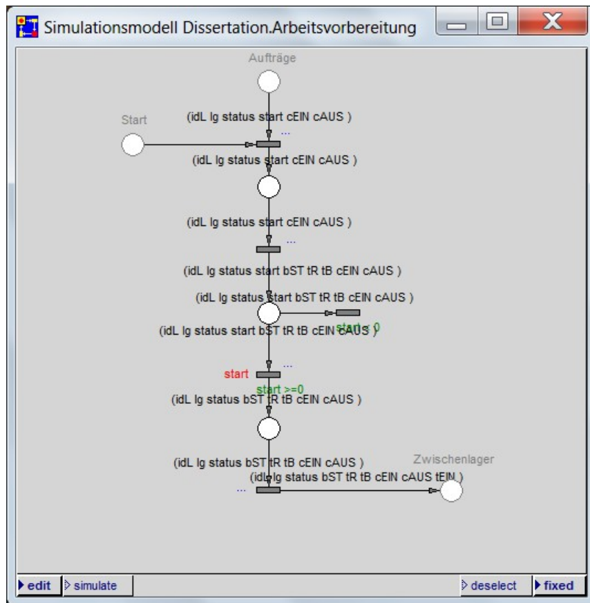
Abbildung 76: Ablaufebene des Moduls Arbeitsvorbereitung des Simulationsmodells Dissertation
