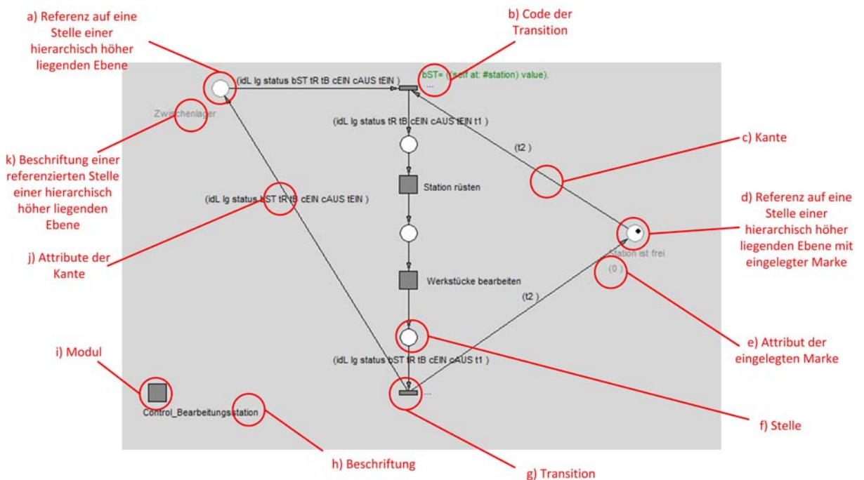
Abbildung 21: In PACE verwendete Elemente
