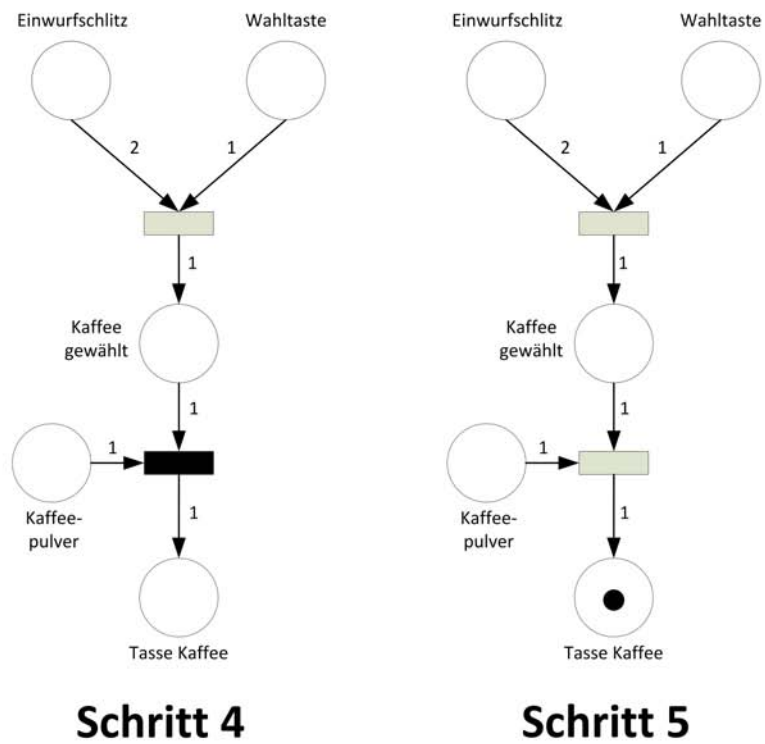
Abbildung 13: Markenspiel im dynamischen Petrinetz-Graphen eines S/T-Netzes
