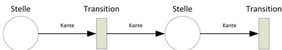
Abbildung 6: Nach den Regeln der statischen Syntax kombinierte Netzelemente
