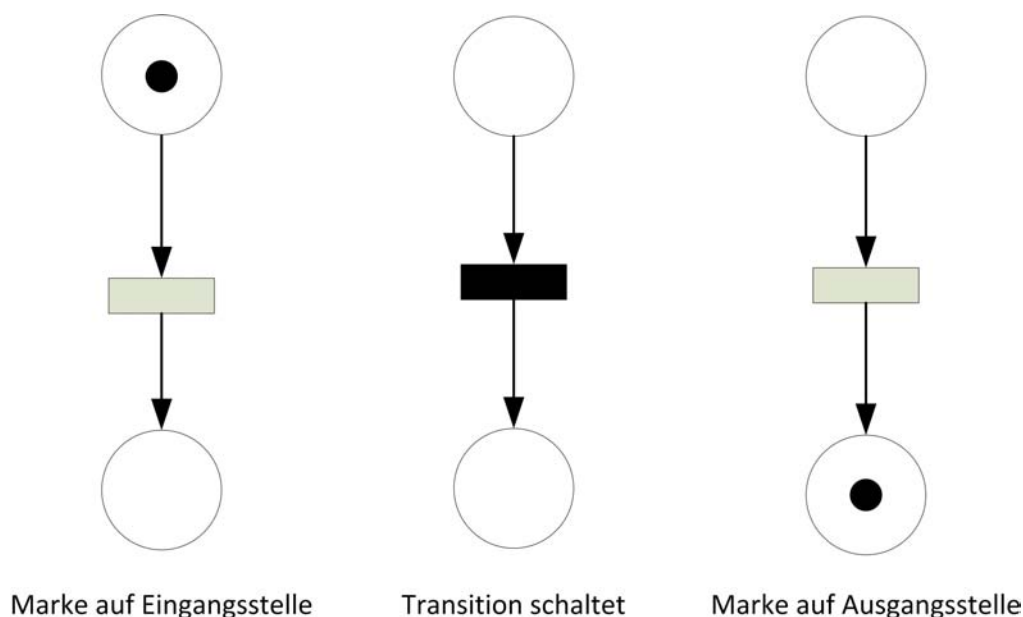
Abbildung 8: Markenspiel eines dynamischen Petrinetz-Graphen
