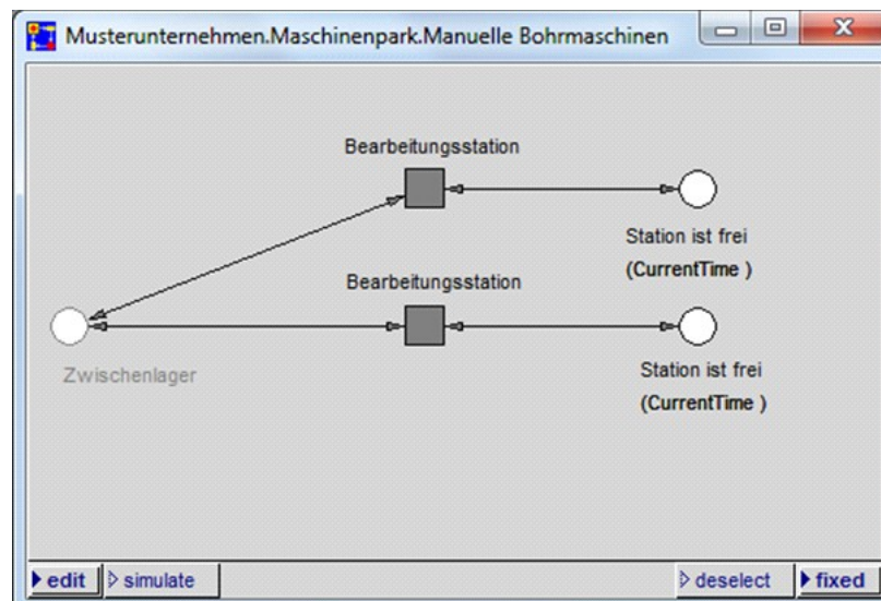
Abbildung 48: Angepasste Kategorie Manuelle Bohrmaschinen
