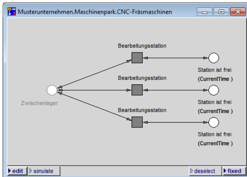
Abbildung 46: Angepasste Kategorie CNC-Fräsmaschinen
