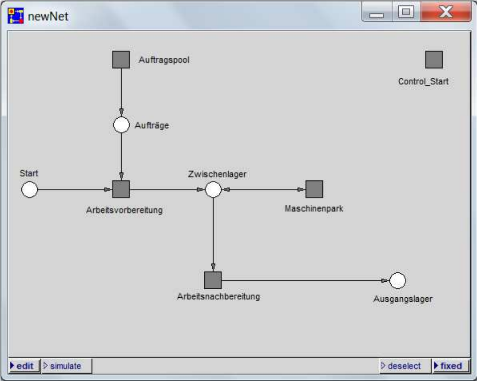
Abbildung 8: Elemente des Basisbausteins (1)
