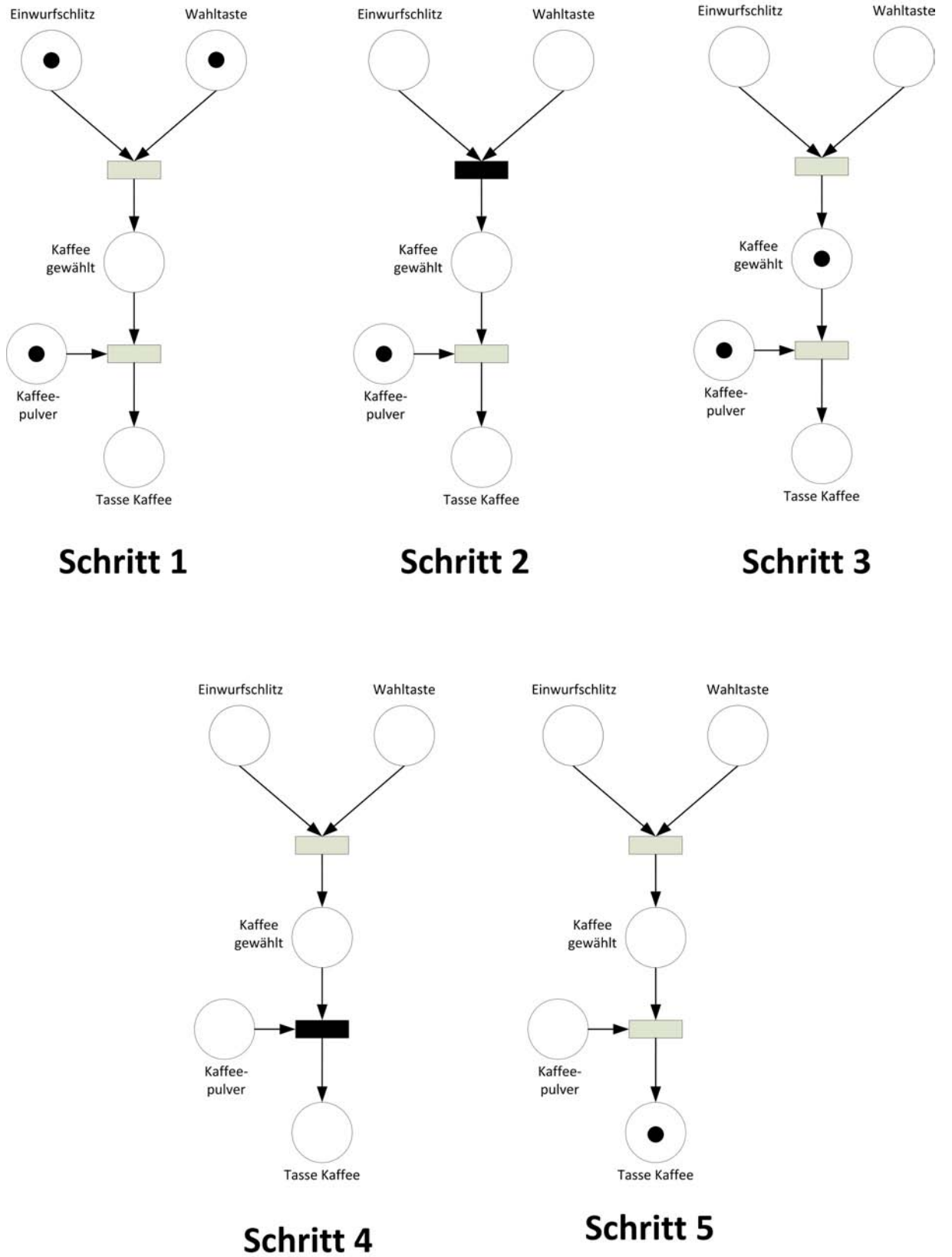
Abbildung 11: Markenspiel im dynamischen Petrinetz-Graphen eines B/E-Netzes
