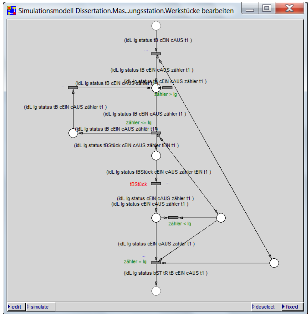
Abbildung 79: Ablaufebene des Moduls Werkstücke bearbeiten des Simulationsmodells Dissertation
