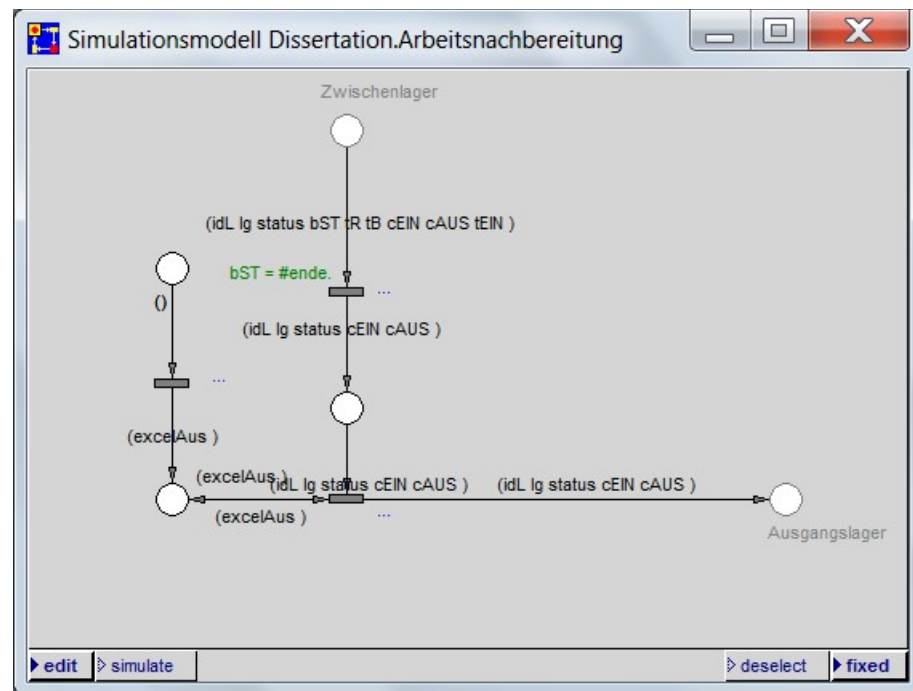
Abbildung 81: Ablaufebene des Moduls Arbeitsnachbereitung des Simulationsmodells Dissertation
