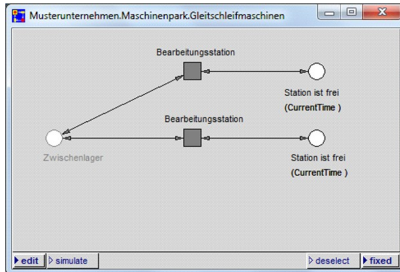
Abbildung 51: Angepasste Kategorie Gleitschleifmaschinen
