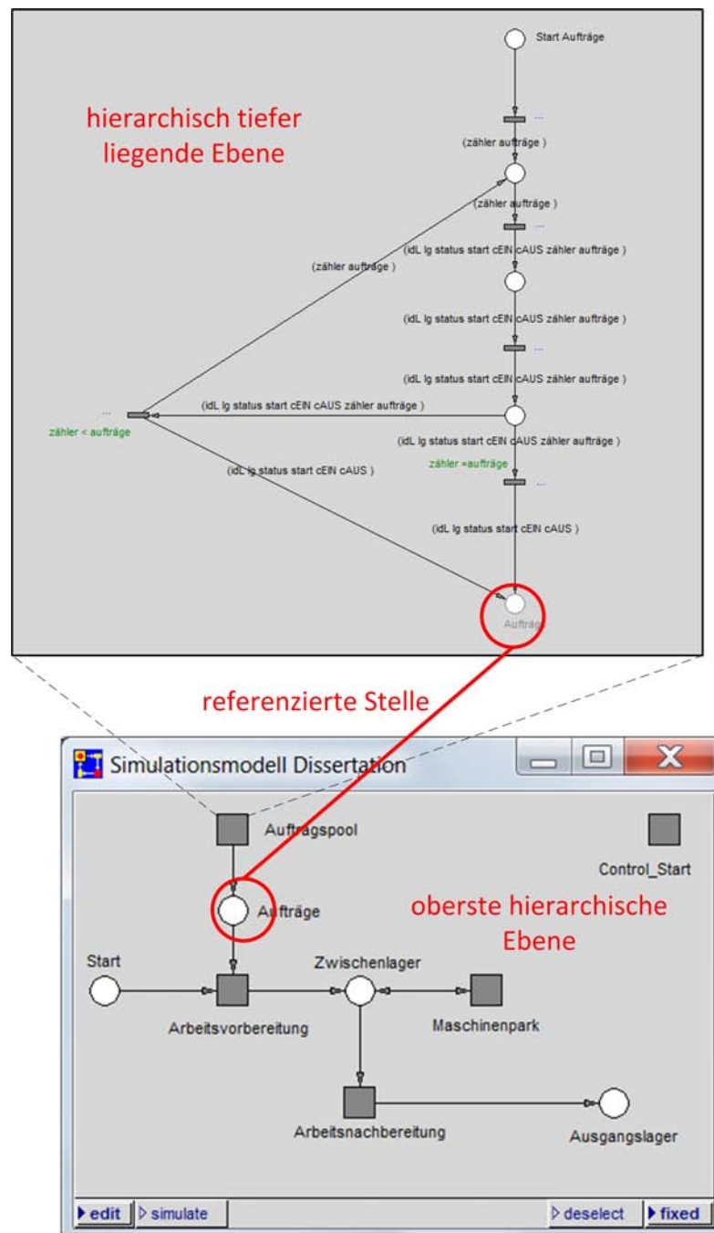
Abbildung 22: Prinzip der Hierarchisierung mittels Modulen in PACE
