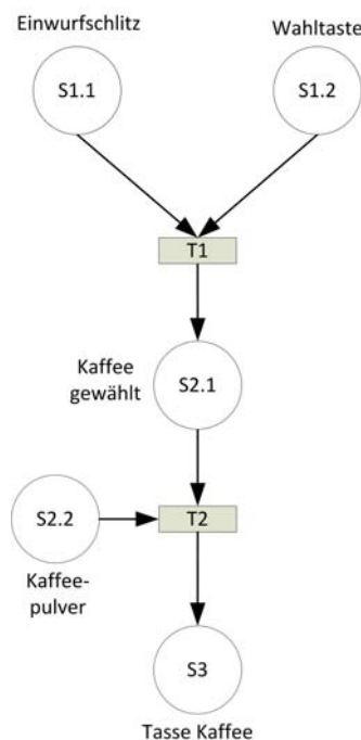
Abbildung 10: Statischer Petrinetz-Graph des Beispiels
