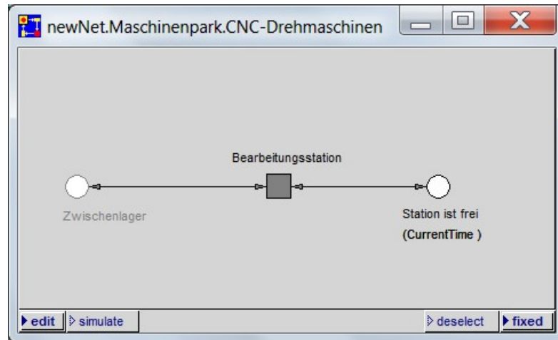
Abbildung 30: Hierarchisch tiefer liegende Ebene einer der Kategorien von Bearbeitungsstationen
