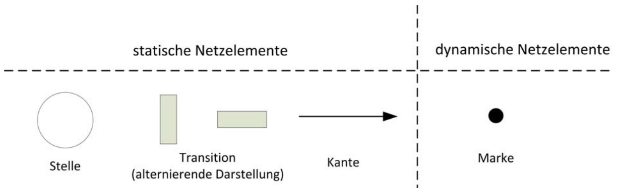
Abbildung 5: Netzelemente der graphischen Notation der Modellierungssprache Petrinetze
