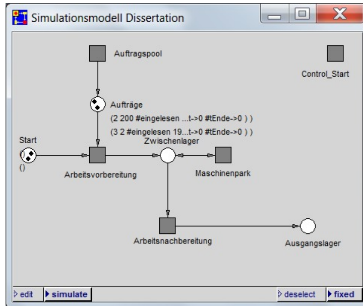
Abbildung 69: Entpackter Basisbaustein mit den Auftragsmarken
