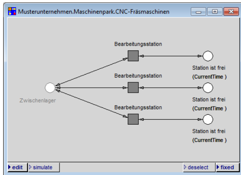
Abbildung 73: 3. Objektebene des Simulationsmodells Musterunternehmen
