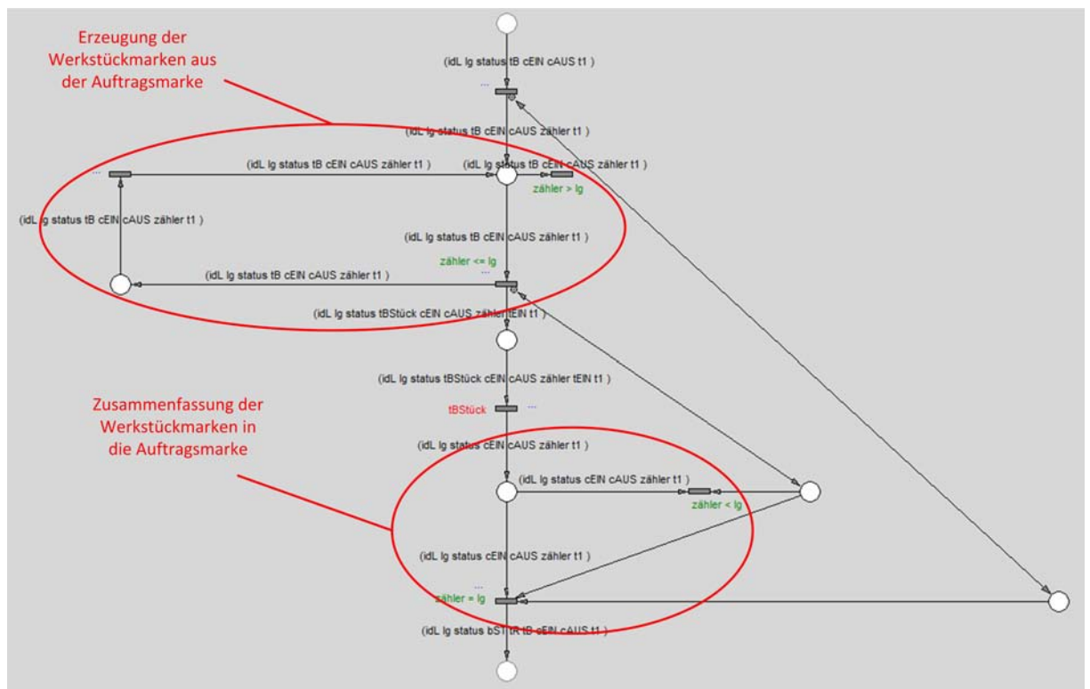
Abbildung 70: Erzeugung der Werkstückmarken sowie Zusammenfassung in die Auftragsmarke im Modul Werkstück bearbeiten
