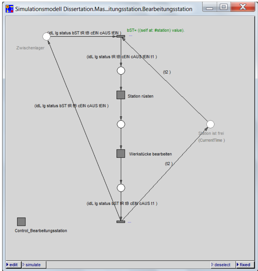
Abbildung 77: Ablaufebene des Moduls Bearbeitungsstation des Simulationsmodells Dissertation
