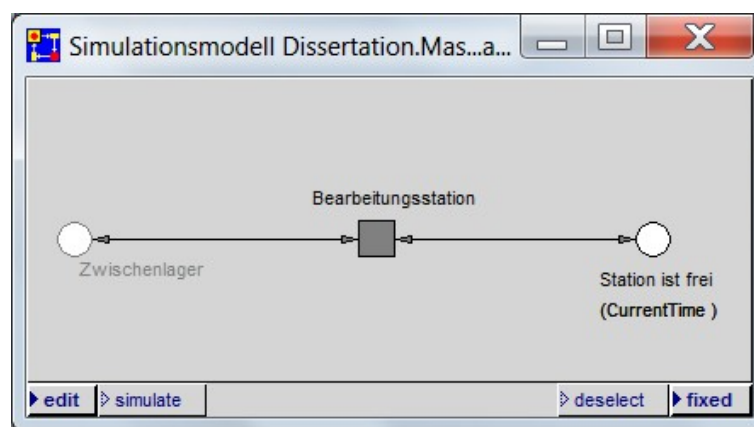
Abbildung 26: PACE-Baustein Bearbeitungsstation
