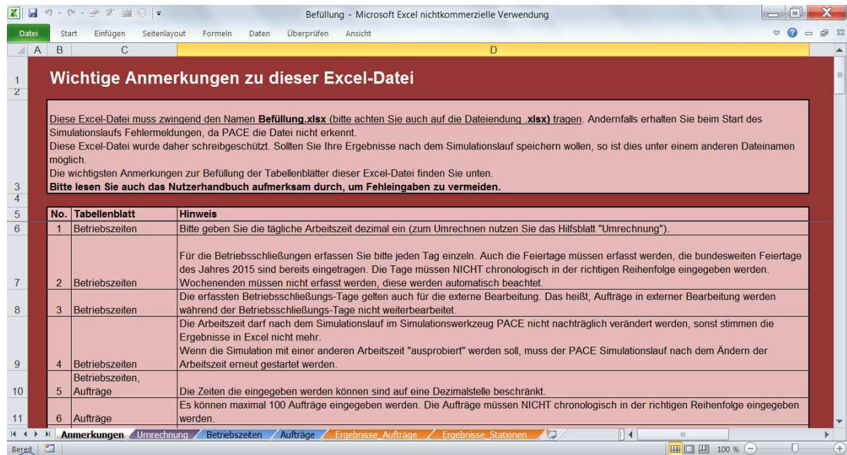
Abbildung 1: Tabellenblatt Anmerkungen
