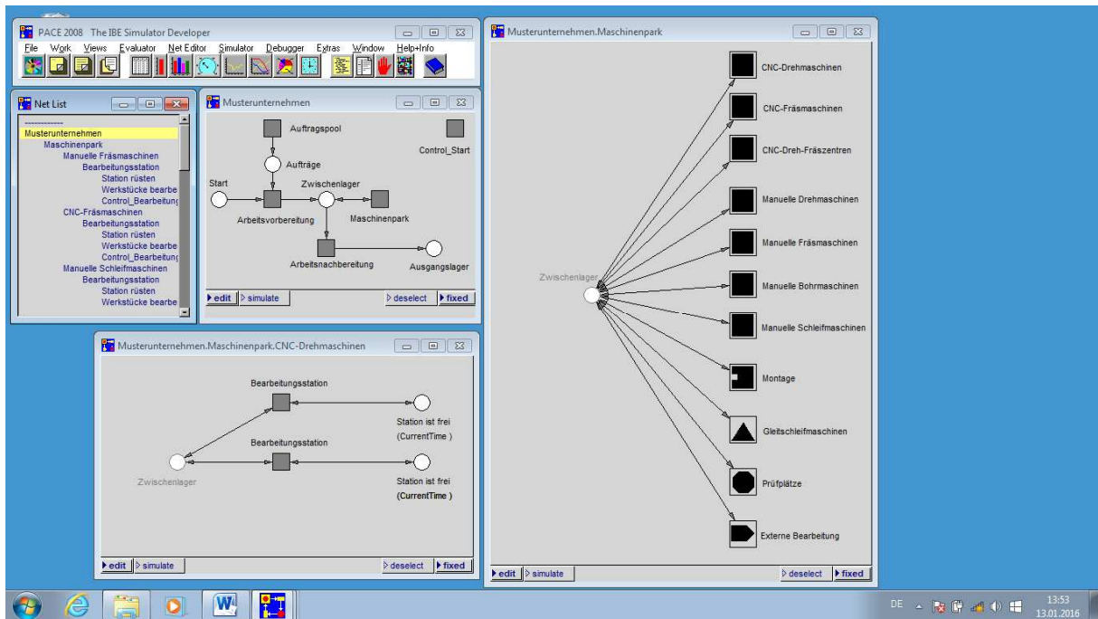
Abbildung 25: Bildschirmansicht (4)
