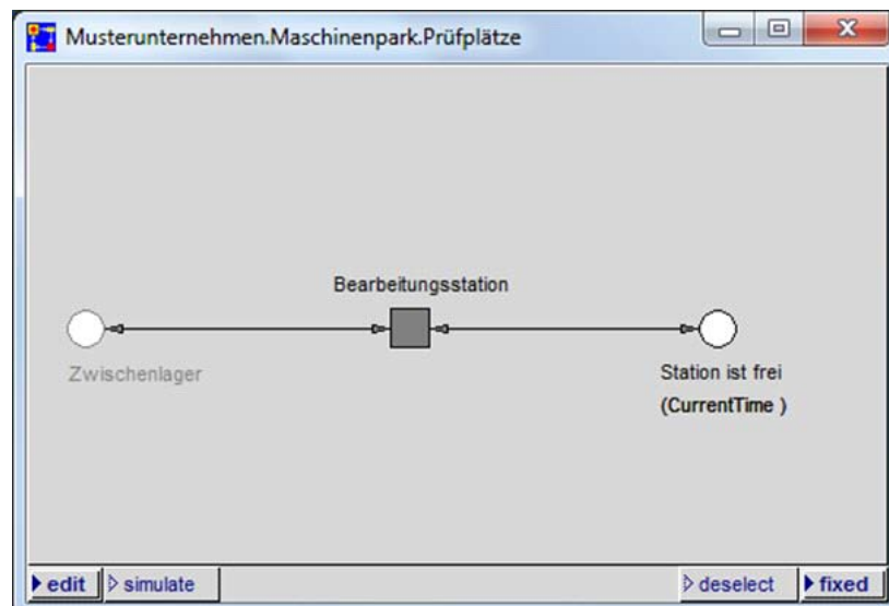
Abbildung 52: Angepasste Kategorie Prüfplätze
