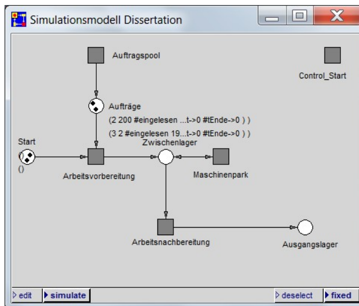
Abbildung 24: Dynamischer Petrinetz-Graph des Simulationsmodells Dissertation auf der obersten hierarchischen Ebene
