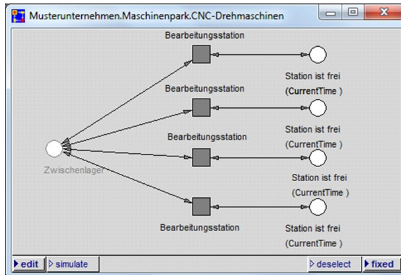
Abbildung 45: Angepasste Kategorie CNC-Drehmaschinen
