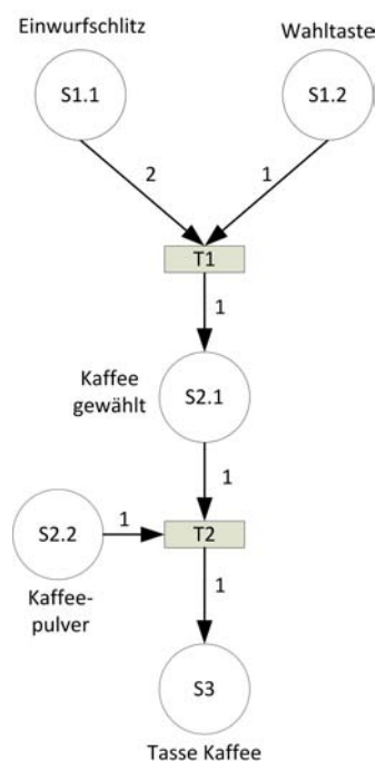
Abbildung 12: Statischer Petrinetz-Graph des abgewandelten Beispiels
