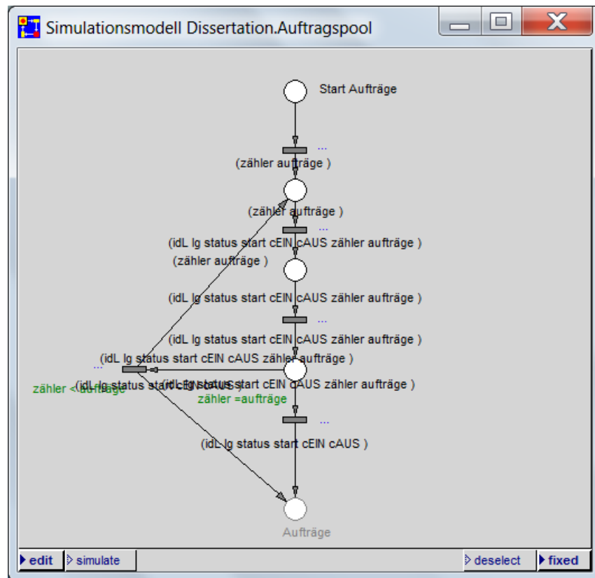
Abbildung 75: Ablaufebene des Moduls Auftragspool des Simulationsmodells Dissertation
