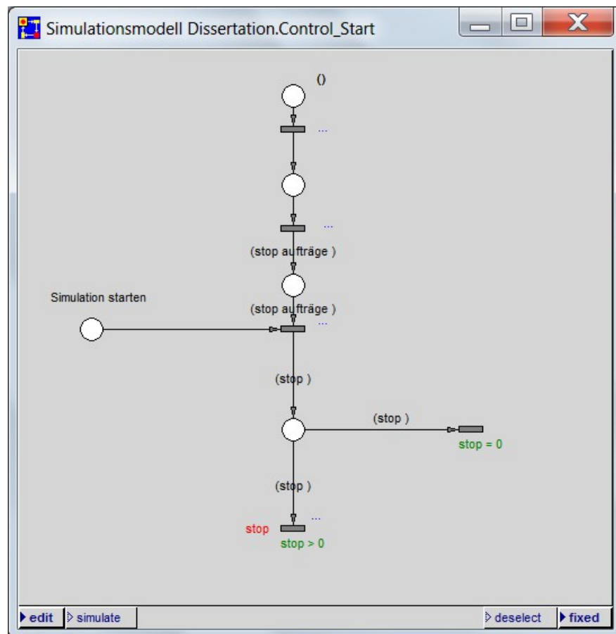
Abbildung 74: Ablaufebene des Moduls Control_Start des Simulationsmodells Dissertation
