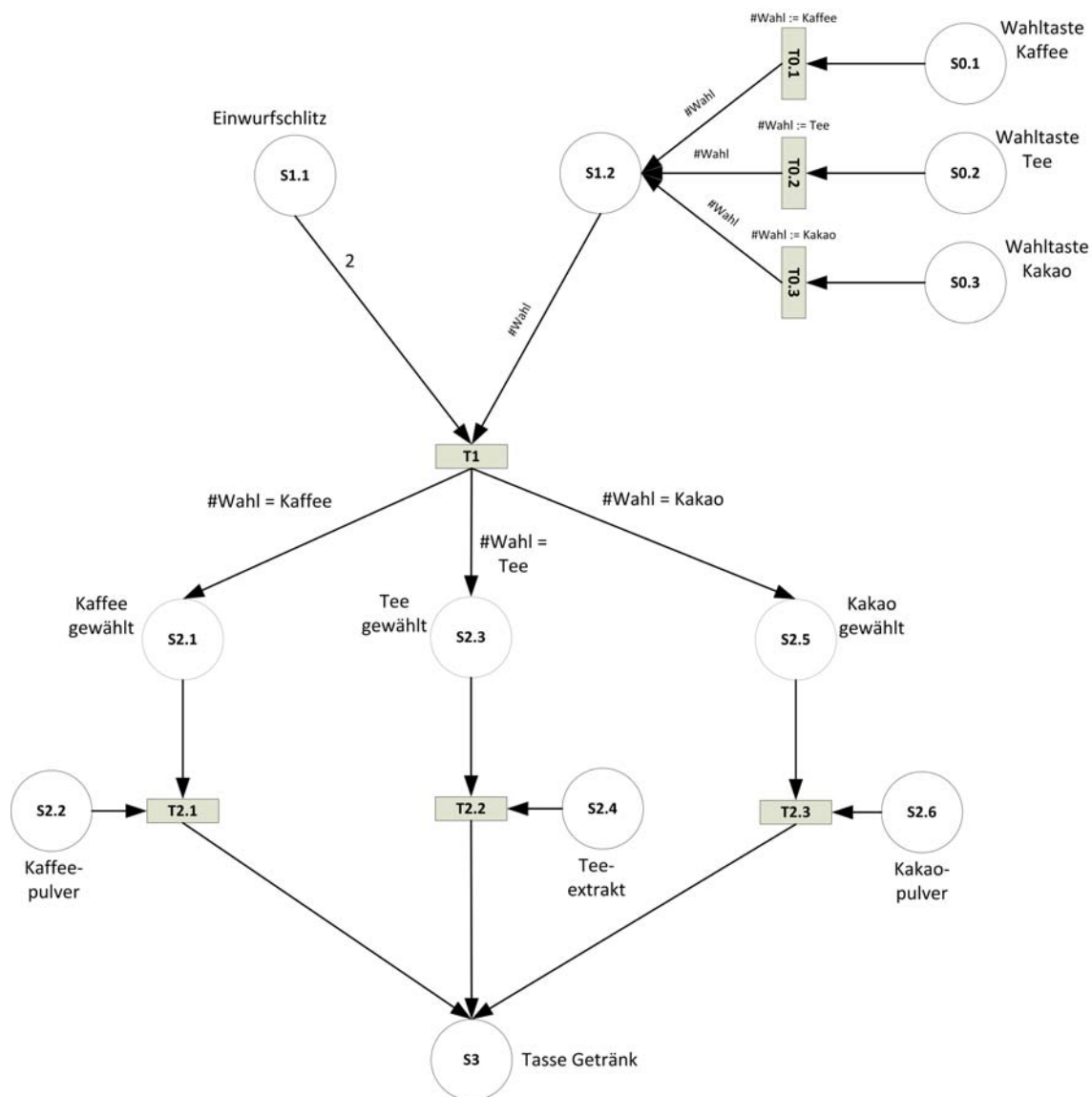
Abbildung 14: Erweiterter statischer Petrinetz-Graph des Beispiels
