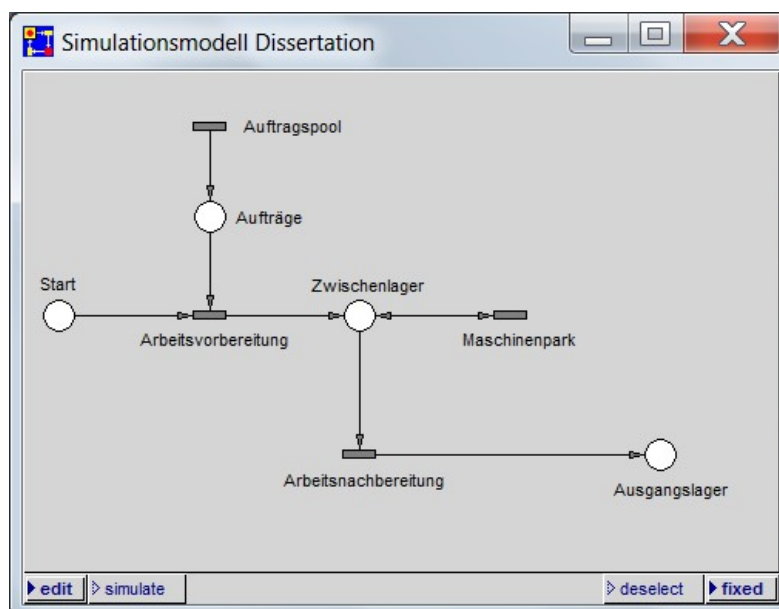
Abbildung 23: Statischer Petrinetz-Graph des Simulationsmodells Dissertation
