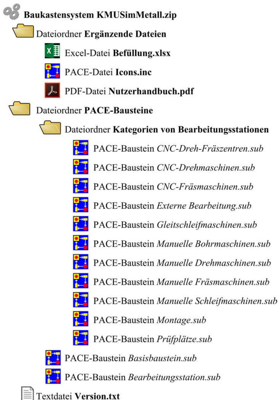
Abbildung 43: Struktur des neuen Baukastensystems KMUSimMetall
