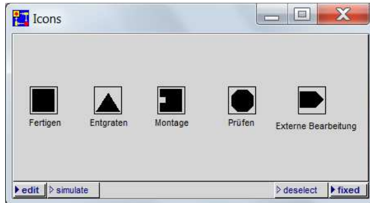
Abbildung 7: Individuelle Icons
