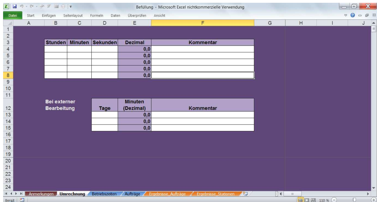
Abbildung 2: Tabellenblatt Umrechnung
