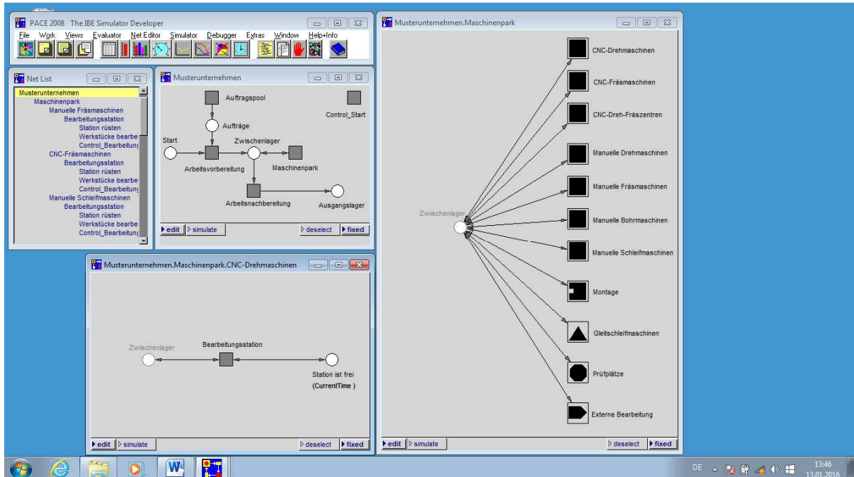
Abbildung 21: Bildschirmansicht (2)
