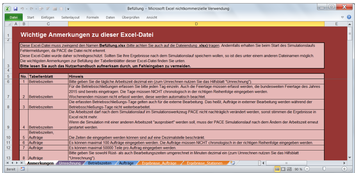
Abbildung 31: Tabellenblatt Anmerkungen
