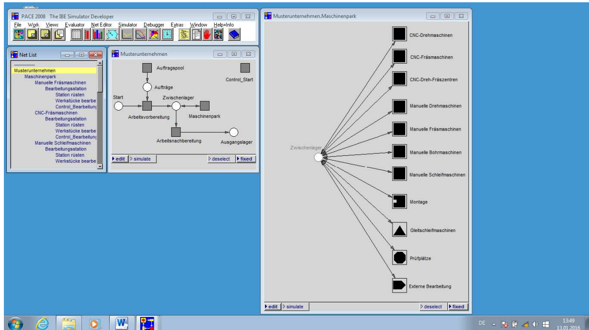
Abbildung 24: Bildschirmansicht (3)
