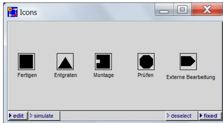
Abbildung 41: Individuelle Icons
