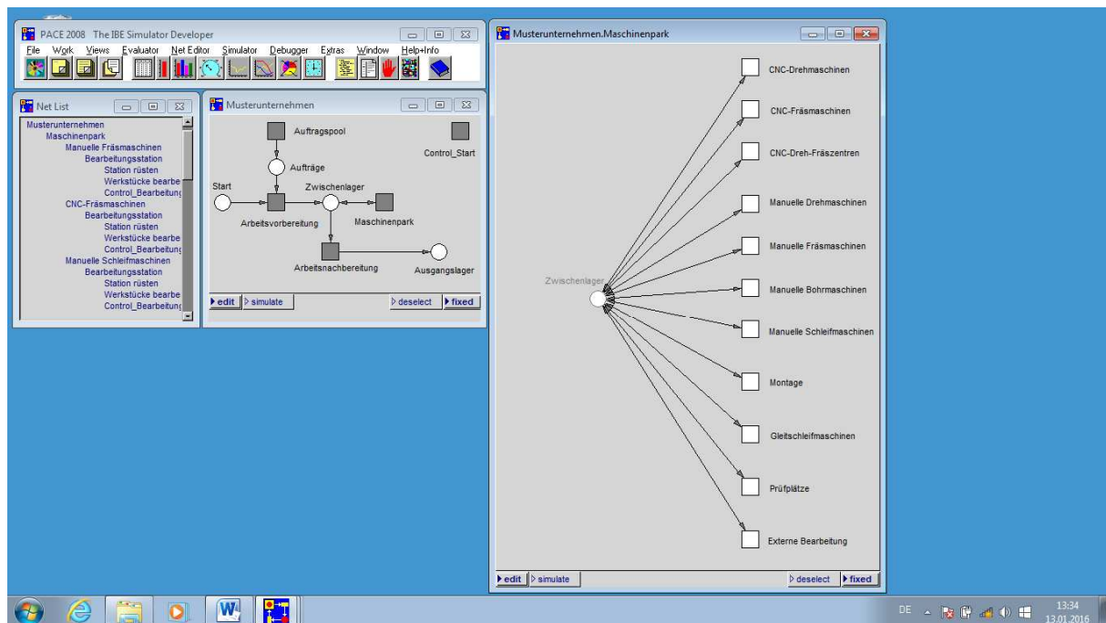
Abbildung 16: Bildschirmansicht (1)
