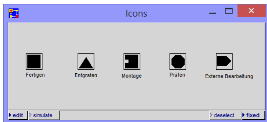
Abbildung 1: Individuelle Icons
