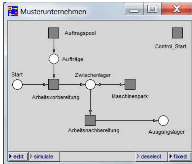
Abbildung 15: Entpackter Basisbaustein
