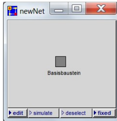
Abbildung 27: PACE-Baustein Basisbaustein
